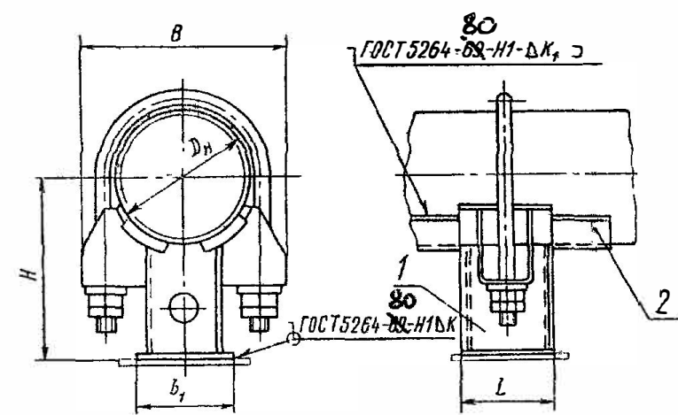
1 — опора однокрутовая; 2 — упор
